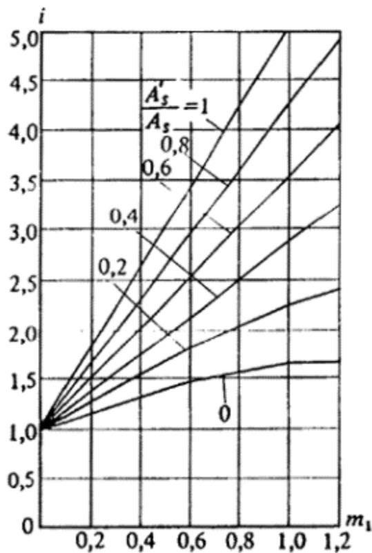
Черт. 2. График значений коэффициента i для вычисления приведенного момента трещинообразования M_{pr} при d = 0,2
