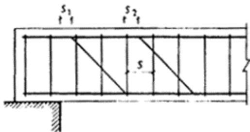
Черт. 8. Расстояния между хомутами и отогнутыми стержнями
