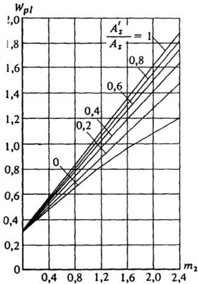
Черт. 3. График значений коэффициента W_{pl} для определения момента появления трещин M_{pl} в изгибаемых элементах прямоугольного сечения при d = 0,1
