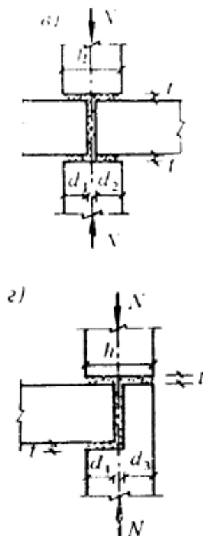
Опорные сечения стен из панелей (блоков)
