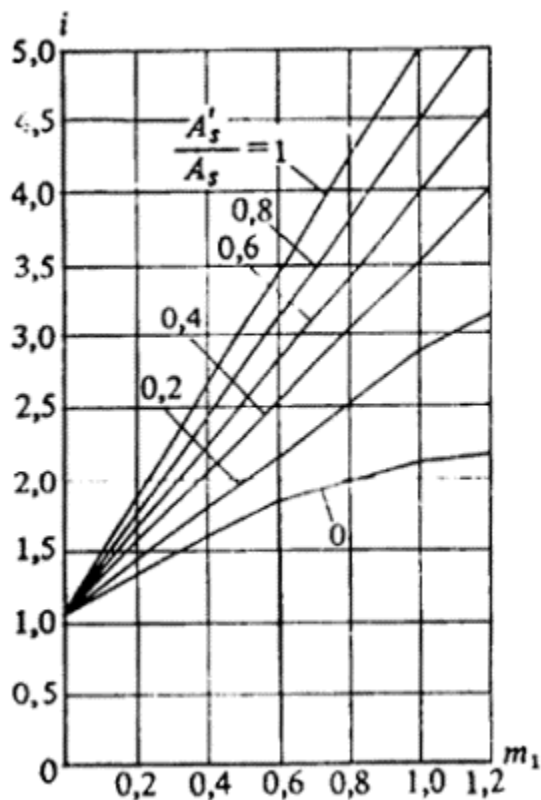
Черт. 1. График значений коэффициента i для вычисления приведенного момента трещинообразования M_{pl} для расчета прогибов изгибаемых элементов прямоугольного сечения при d = 0,1
